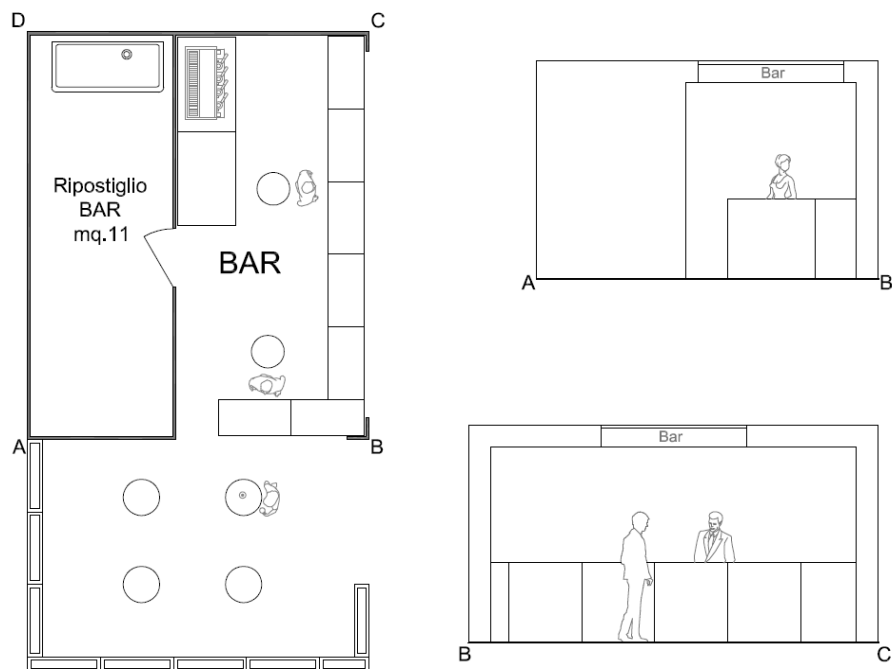
Figura 4 - Particolare Esemplativo Area Bar
