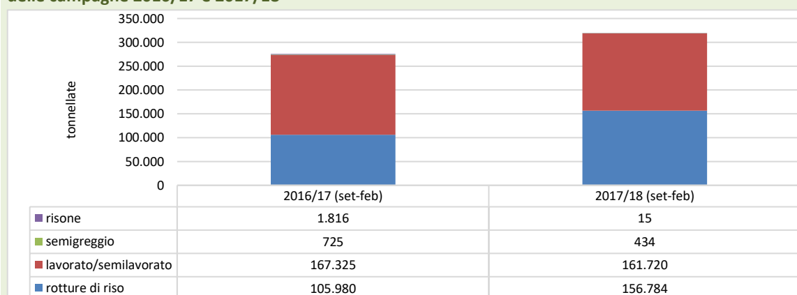
Grafico 2.2: Importazioni comunitarie di riso (tonnellate) dai Paesi EBA nel periodo settembre-febbraio delle campagne 2016/17 e 2017/18
