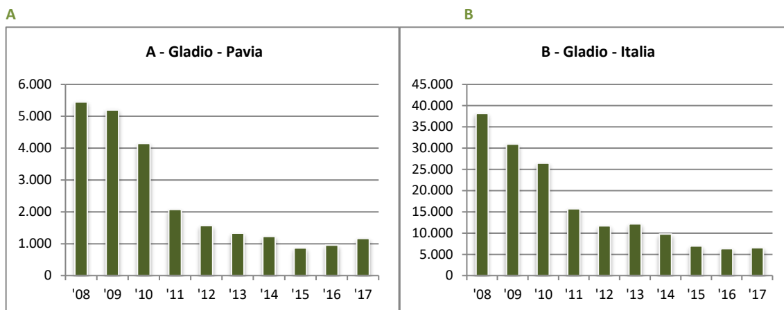
Grafico 1.16: Superficie (.000 ha) investita a riso GLADIO a Pavia (A) e in Italia (B) (2008-2017)
