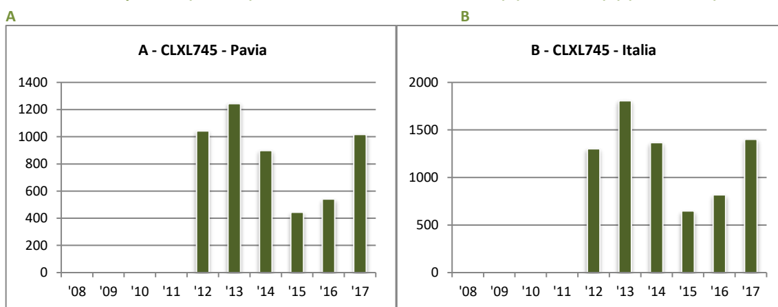
Grafico 1.17: Superficie (.000 ha) investita a riso CLXL745 a Pavia (A) e in Italia (B) (2008-2017)
