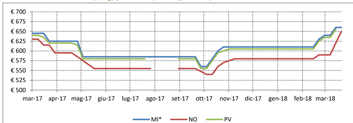
Grafico 1.4: Prezzo medio (€/kg) per CCIAA (franco partenza) Riso lavorato – Lido e similari
