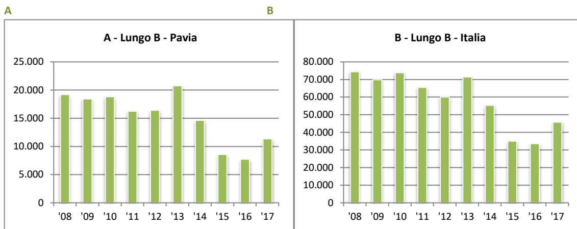
Grafico 1.12: Superficie (.000 ha) investita a riso LUNGO B a Pavia (A) e in Italia (B) (2008-2017)
