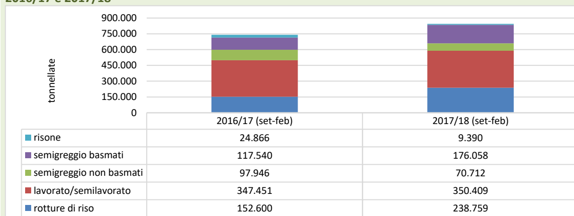
Grafico 2.1: Importazioni comunitarie di riso (tonnellate) nel periodo settembre-febbraio delle campagne 2016/17 e 2017/18
