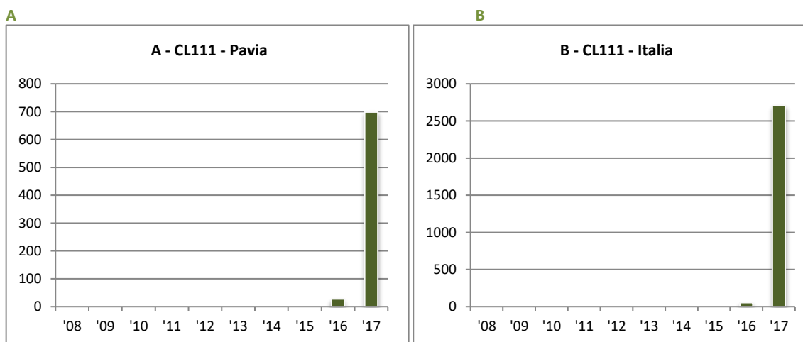
Grafico 1.18: Superficie (.000 ha) investita a riso CL111 a Pavia (A) e in Italia (B) (2008-2017)
