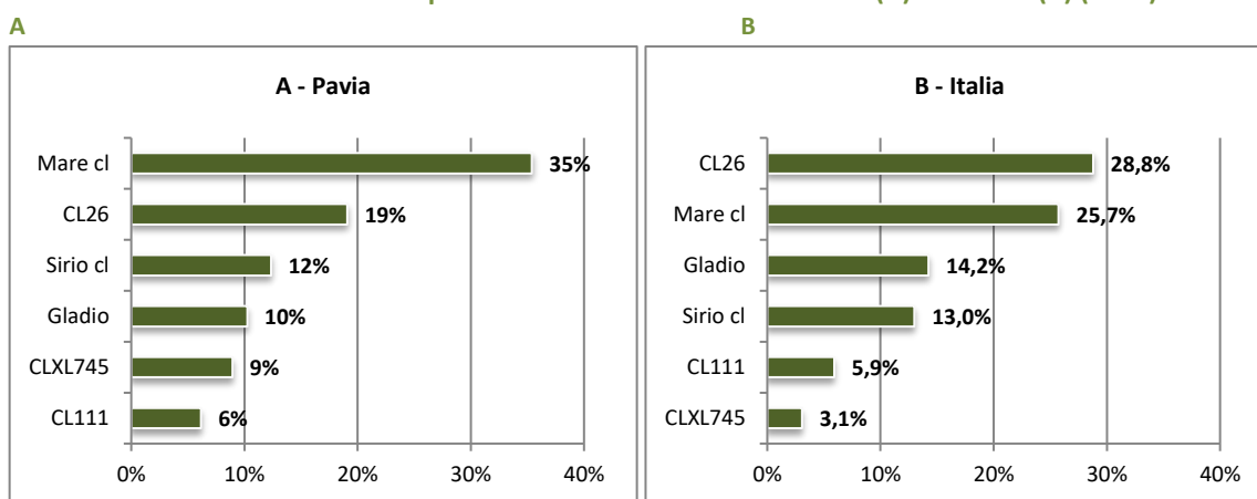
Grafico 1.11: Suddivisione della superficie investita a LUNGO B a Pavia (A) e in Italia (B) (2017)
