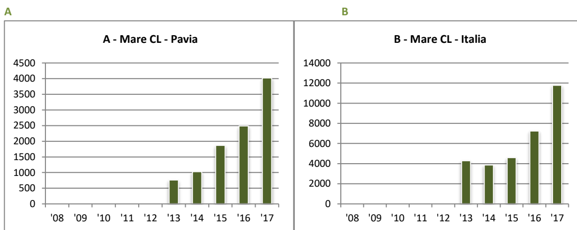
Grafico 1.13: Superficie (.000 ha) investita a riso MARE CL a Pavia (A) e in Italia (B) (2008-2017)
